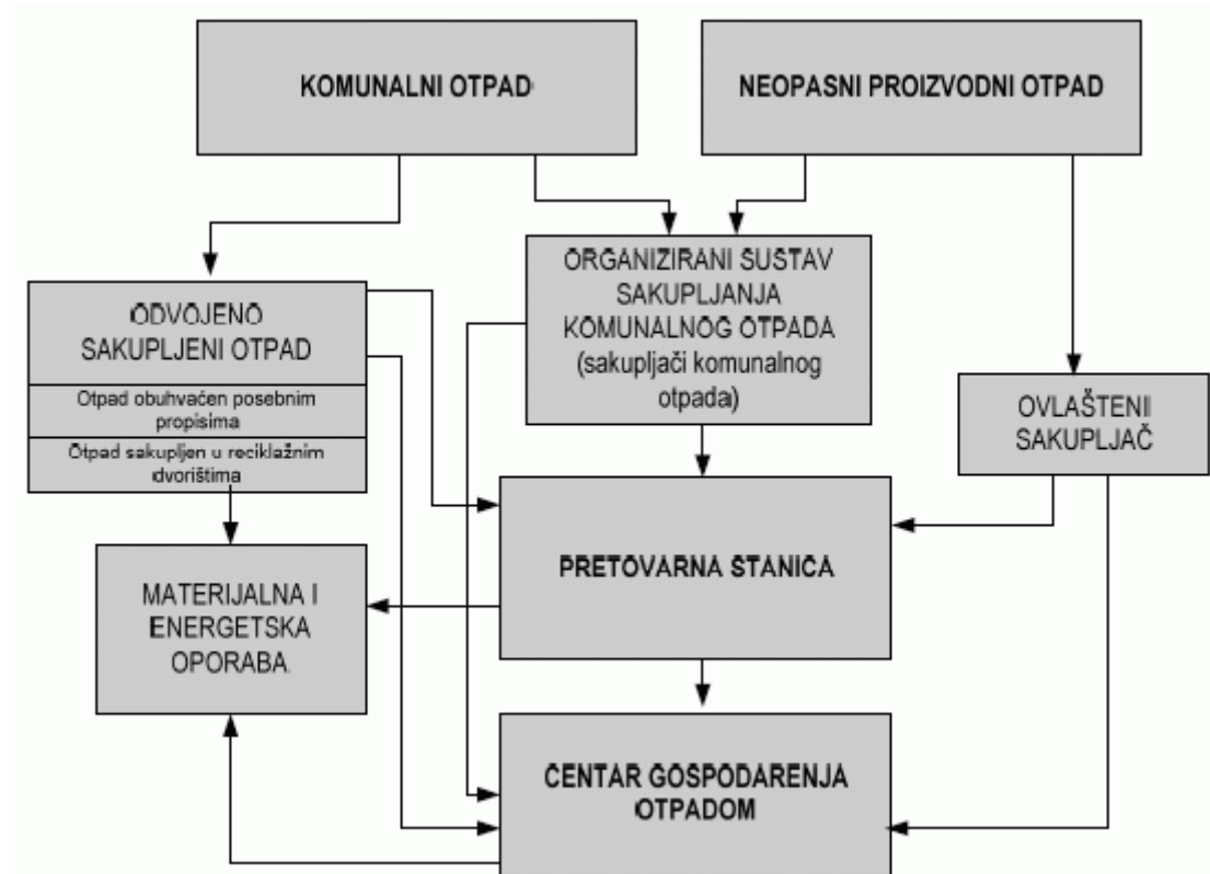
SLIKA 17. Blok – dijagram sustava gospodarenja komunalnim i neopasnim proizvodnim otpadom
