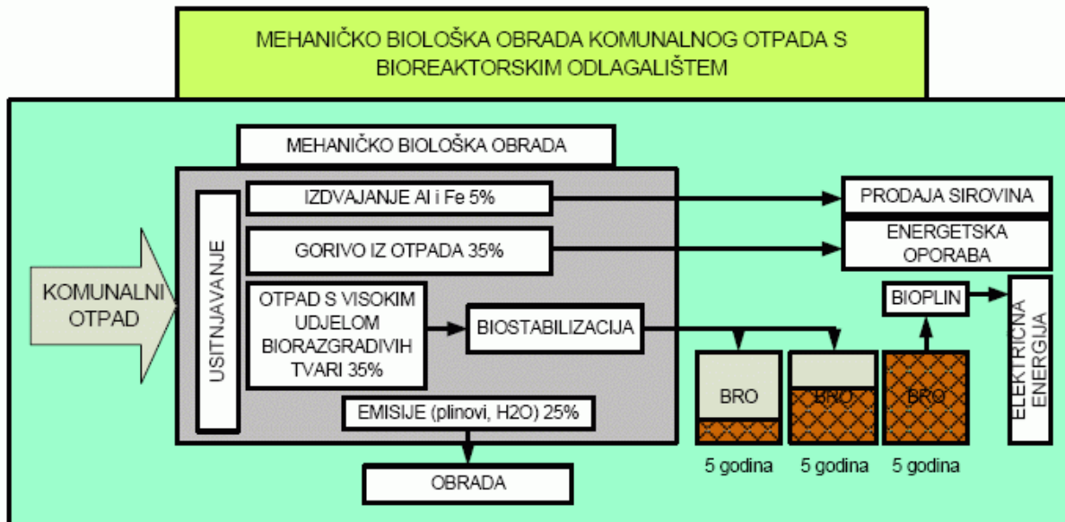
SLIKA 25. MBO s bioreaktorskim odlagalištem
